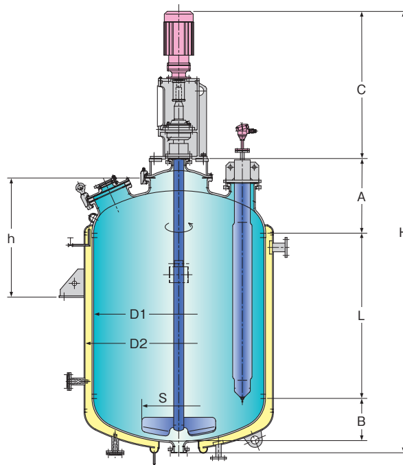
反応機 標準寸法表
